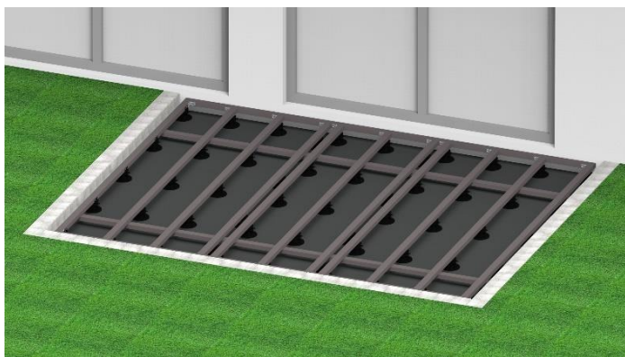
Bild 10. Mit mindestens 2 untergeschraubten Unterkonstruktionen kann eine einfache und stabile Aussteifung erzielt werden.
