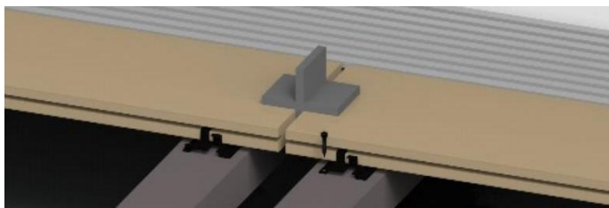
Bild 16. Mit handelsüblichen Abstandhaltern können gleichmäßige Fugenabstände an den Längsstößen der WPC-Dielen sichergestellt werden. Die Abstände sind von der Verlegetemperatur der WPC-Dielen abhängig.
