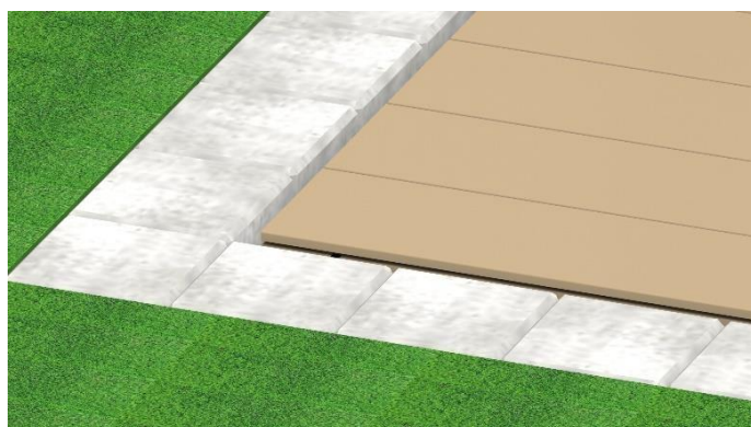
Bild 31. Der Fugenabstand an der letzten WPC-Deile beträgt bei richtiger Montage ca. 20 mm zur Steinkante und der Abstand der Unterkonstruktion beträgt ca. 10 mm.
