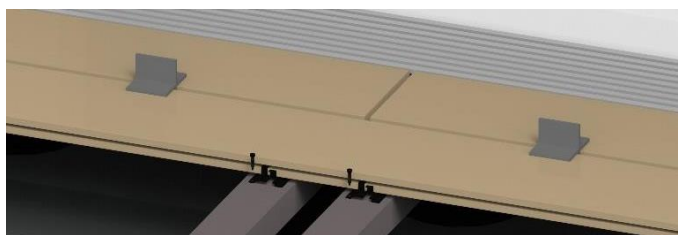
Bild 17. Mit Abstandshaltern kann einfach eine ca. 1 mm größere Fuge sichergestellt werden als die Befestigungssysteme vorgeben.
