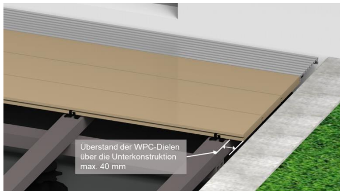
Bild 24. An den äußeren Unterkonstruktionen darf der Überstand der WPC-Dielen max. 40 mm betragen. Der Fugenabstand an den Dielenenden zu festen Bauteilen muss 20 mm betragen.
