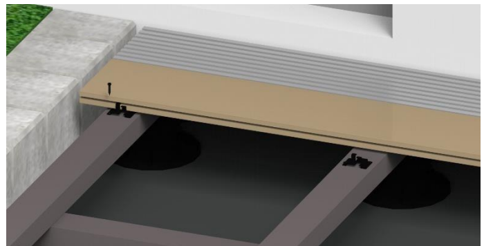
Bild 22. Die WPC-Diele wird mit dem notwendigen Abstand ausgerichtet und die Befestigungsclips unter die Dielen geschoben.
