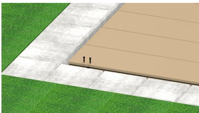
Bild 30. Die Anfangs-/Endclips werden mit den beiliegenden Schrauben auf der Unterkonstruktion befestigt.
