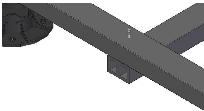
Bild 11. Die Verschraubung erfolgt von oben mit nicht rostenden Edelstahlschrauben. Wenn möglich sollte die Verschraubung in den Steg der unteren Unterkonstruktion eingeschraubt werden.
