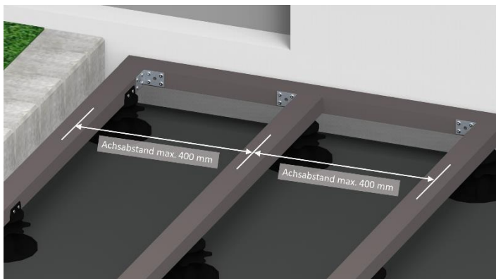
Bild 8. Der Achsabstand der Unterkonstruktionen darf 400 mm nicht überschreiten.
