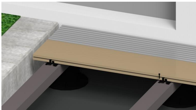
Bild 23. Mit je 1 Edelstahlschraube 4,2 x 22 mm wird der Befestigungsclip auf der Unterkonstruktion verschraubt. Bitte beachten Sie das die Verschraubung mit dem richtigen Drehmoment erfolgt (ca. 3,6 Nm).
